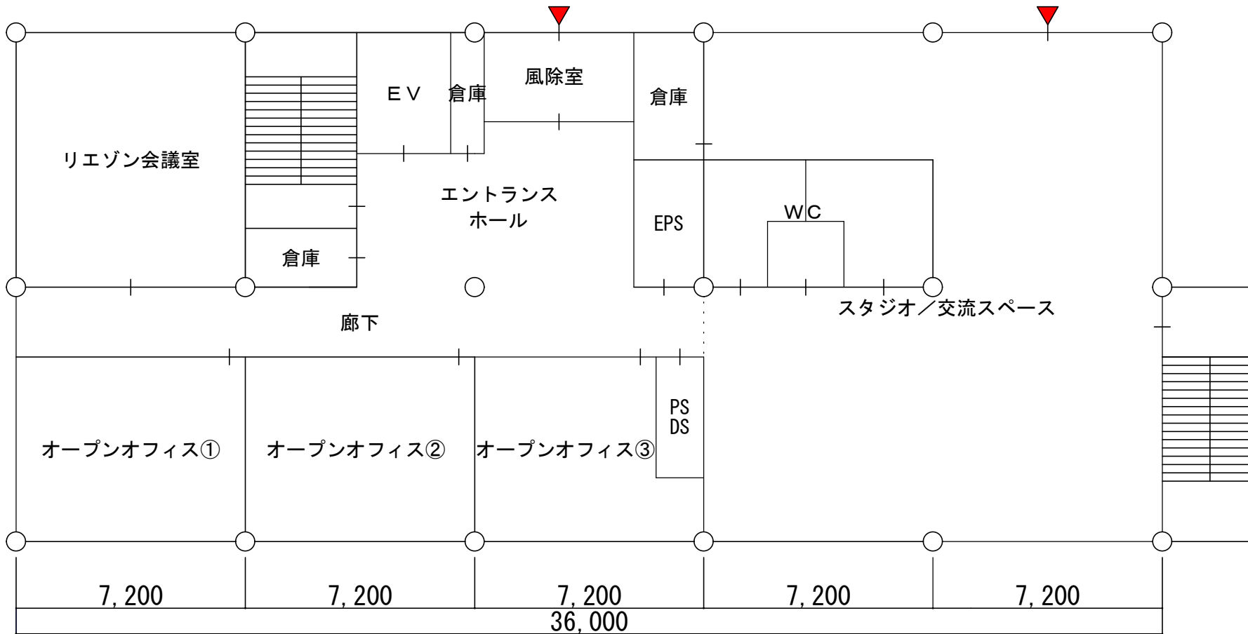
2階平面図
